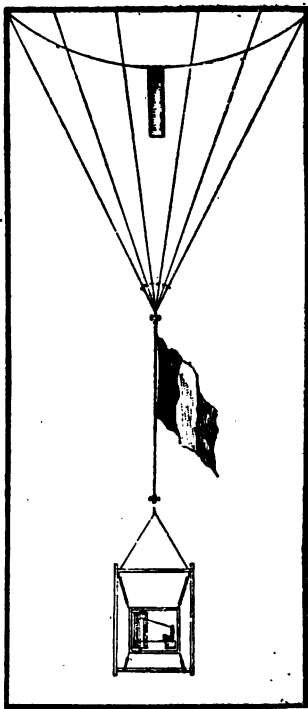
Disposition des enregistreurs français et de leur suspension élastique.
